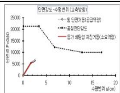
교각 연성도 평가
